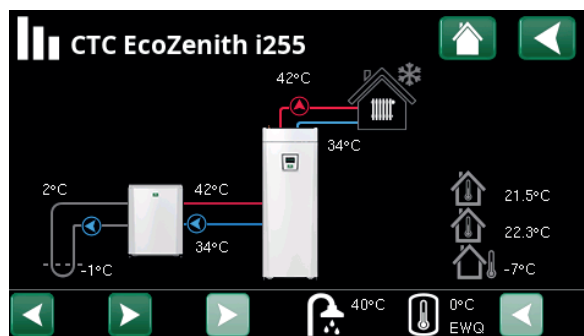
Der Bildschirm enthält die Betriebsdaten mit angeschlossener CTC EcoPart Wärmepumpe.
