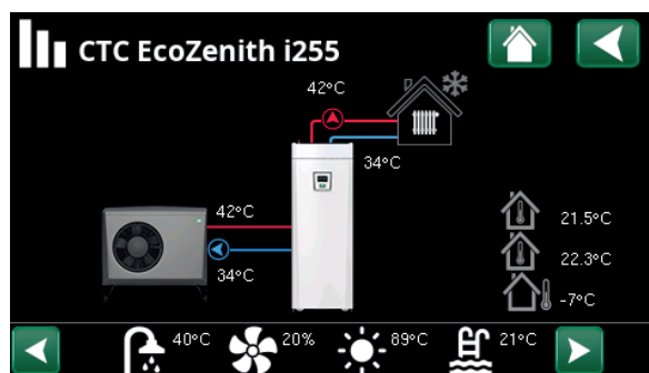
Der Bildschirm zeigt die Betriebsdaten mit angeschlossener CTC EcoAir Wärmepumpe.
