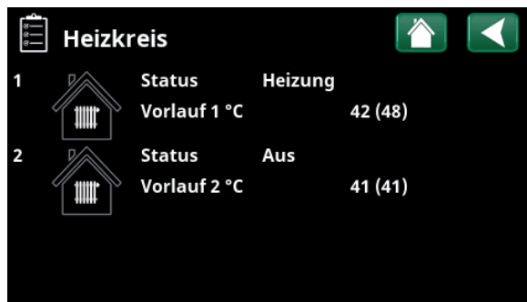
Menü „Betriebsinfo Heizkreis“ Im Menü werden die aktuellen Temperaturen und der Status festgelegter Heizkreise angezeigt.
