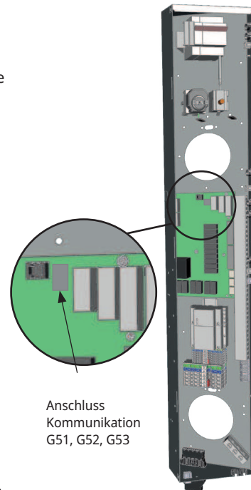
Anschlusskasten EcoZenith
