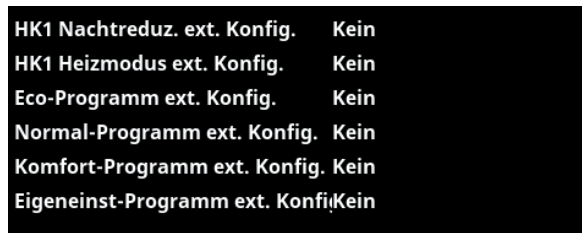
Ausschnitt aus dem Menü „Fachmann/Definieren/Heizkreis“. In den Menüleisten „Programm Eco / Normal / Komfort / Eigene Einstellungen ...“ wird der Normalbetriebs-Modus durch das externe Steuersignal („Schließer (NO)“ oder „Öffner (NC)“) angezeigt.
