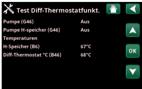
Menü: „Fachmann/Service/Funktionstest/Diff Thermostat“.
