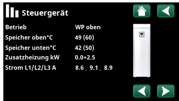
Menü: „Betriebsinfo/Steuerung“ Klicken Sie auf die Pfeile oder wischen Sie, um zwischen Steuergerät und Wärmepumpe umzuschalten.
