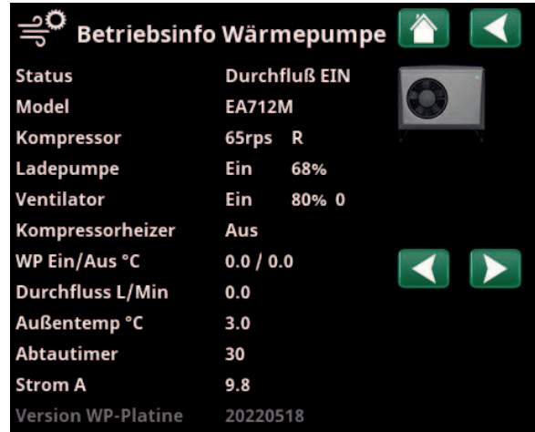
Menü: Betriebsdaten Wärmepumpe.
