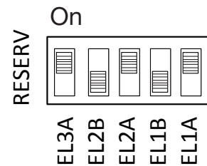
Beispiel für 1,2+0,6+0,3 = 2,1 kW 3~
