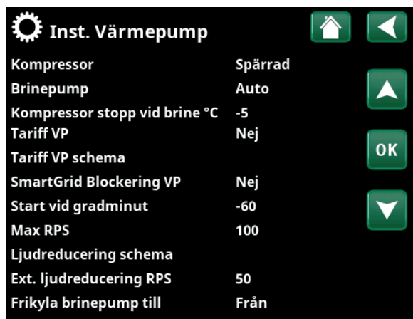
Meny "Avancerat/Inställningar/Värmepump".
