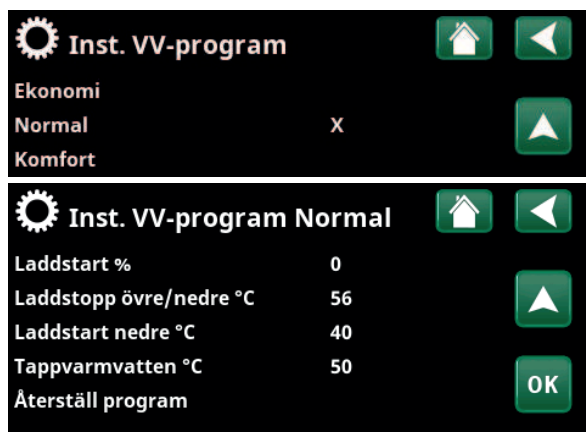
Menyer "Avancerat/Inställningar/Varmvatten/VV-program".
