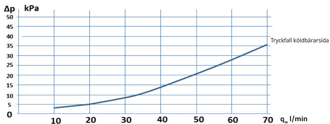
CTC GSi 616
