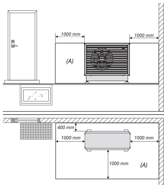
Varnostno območje toplotne črpalke (A) pri namestitvi v kot.
