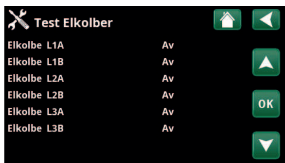
Meny «Avansert/Service/Funksjonstest/Elkolber».
