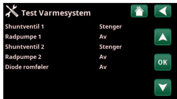
Meny «Avansert/Service/Funksjonstest/Varmesystem».
