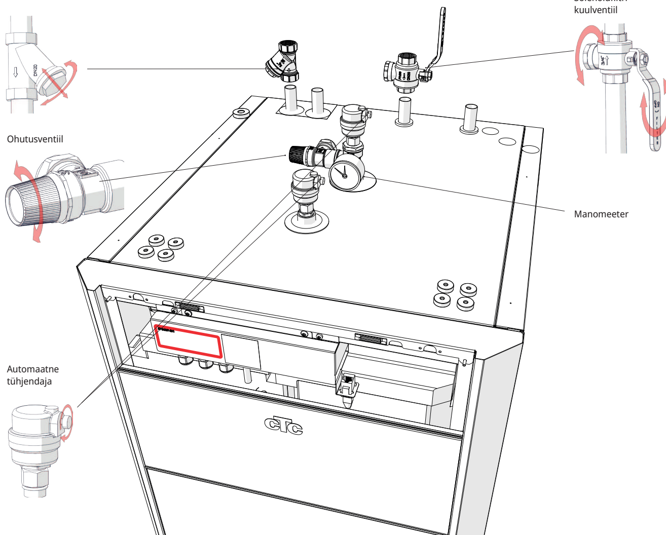
Kraanivee mustusefilter
