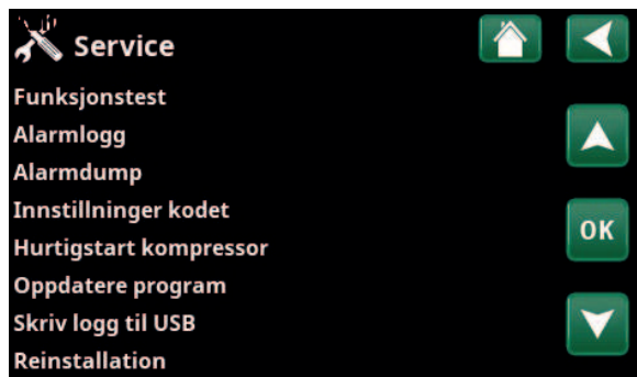
Meny «Avansert/Service» (EcoZenith i360).
