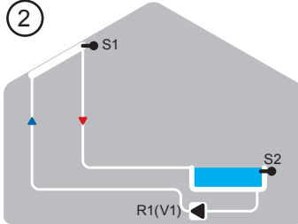
Solar mit Pool
