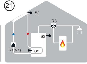
Solar + Thermostat und Ventil
