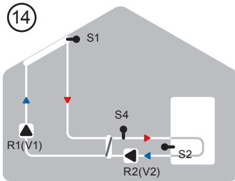
Solar + Wärmetauscher
