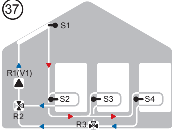
Solar mit 3 Speichern und 3 Ventilen
