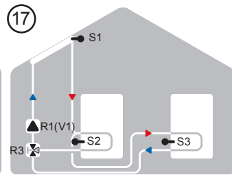
Solar + 2. Speicher mit Ventil
