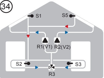
Solar mit 2 Kollektoren, 2 Speichern und 2 Pumpen
