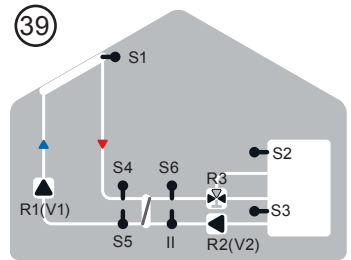
Solar mit Wärmetauscher, 2-Zonenspeicher und Ventil
