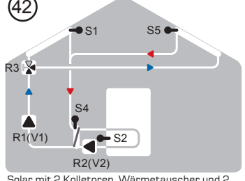
Solar mit 2 Kollektoren, Wärmetauscher und 2 Pumpen
