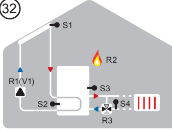
Solar mit Thermostat und Rücklaufanhebung
