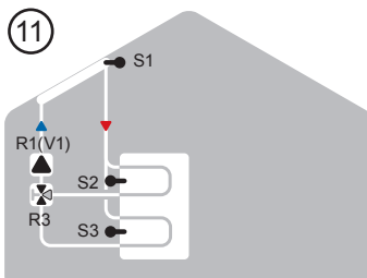
Solar + 2 Zonenspeicher
