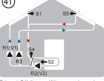
Solar mit 2 Kollektoren, Wärmetauscher und 3 Pumpen
