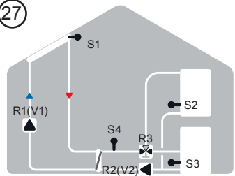
Solar mit Wärmetauscher, 2 Speichern und Ventil
