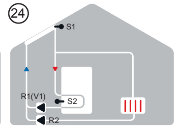
Solar + Kühlung 2
