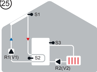
Solar + Kühlung 3
