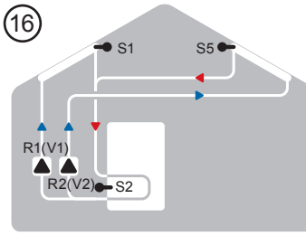
Solar + 2 Kollektoren + 2 Pumpen
