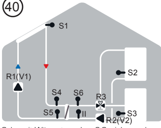
Solar mit Wärmetauscher, 2 Speicher und Ventil
