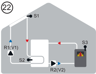
Solar + Feststoffkessel
