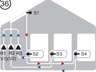
Solar mit 3 Speichern und 3 Pumpen
