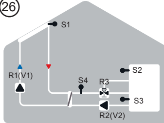
Solar mit Wärmetauscher, 2-Zonenspeicher und Ventil
