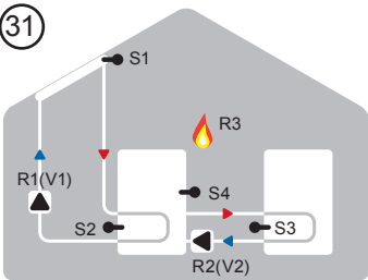
Solar mit Thermostat und Umladung
