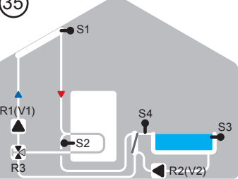
Solar mit Pool, Speicher und Wärmetauscher
