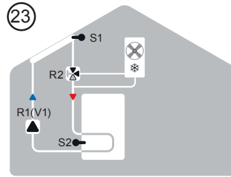
Solar + Kühlung 1
