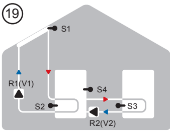
Solar + Umladung
