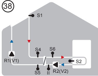
Solar mit Wärmetauscher
