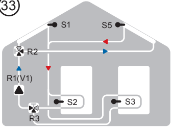
Solar mit 2 Kollektoren, 2 Speichern und 2 Ventilen
