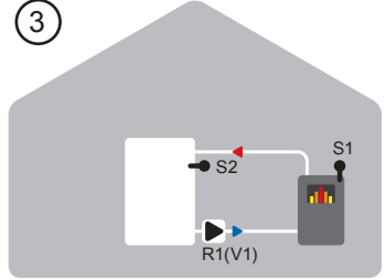
Feststoffkessel mit Speicher
