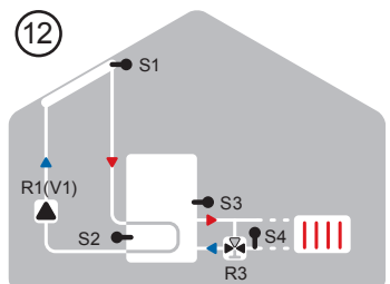
Solar + Rücklaufhebung
