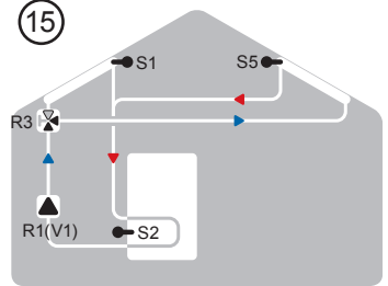
Solar + 2 Kollektoren
