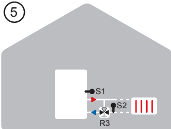
Rücklaufhebung
