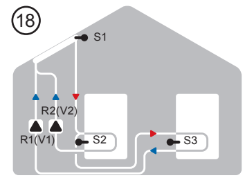
Solar + 2. Speicher + 2 Pumpen
